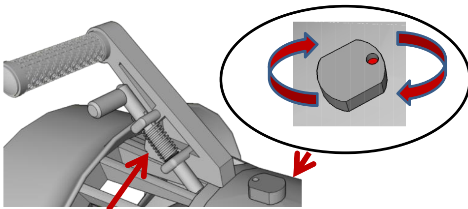
Commande de veille, ressort allongé
